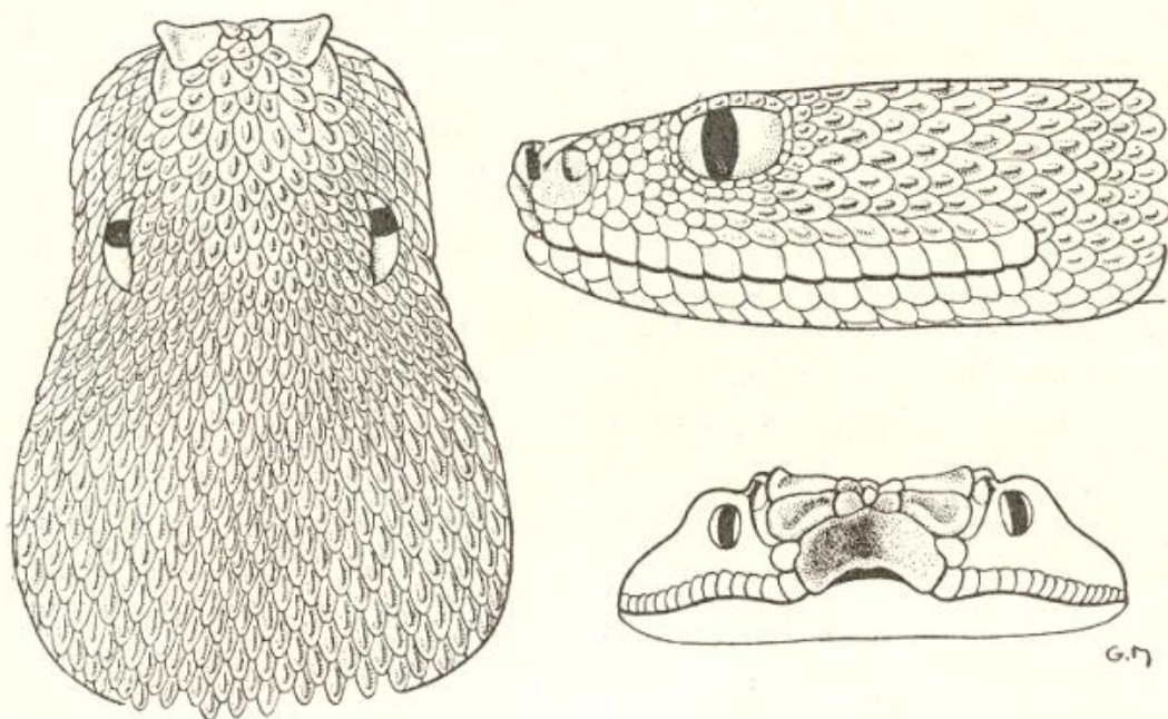
Pseudocerastes latirostris n. sp.
